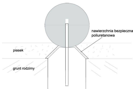
Fundament o szerokości - 5cm średnicy kuli i wysokości kuli
